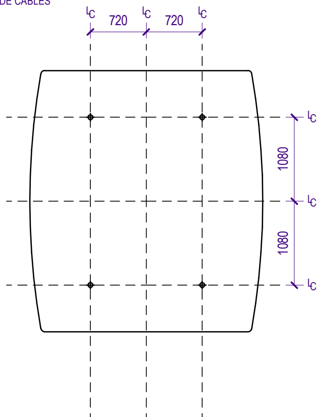
PLANTA DE CENTROS PARA ACOMETIDA DE CABLES
