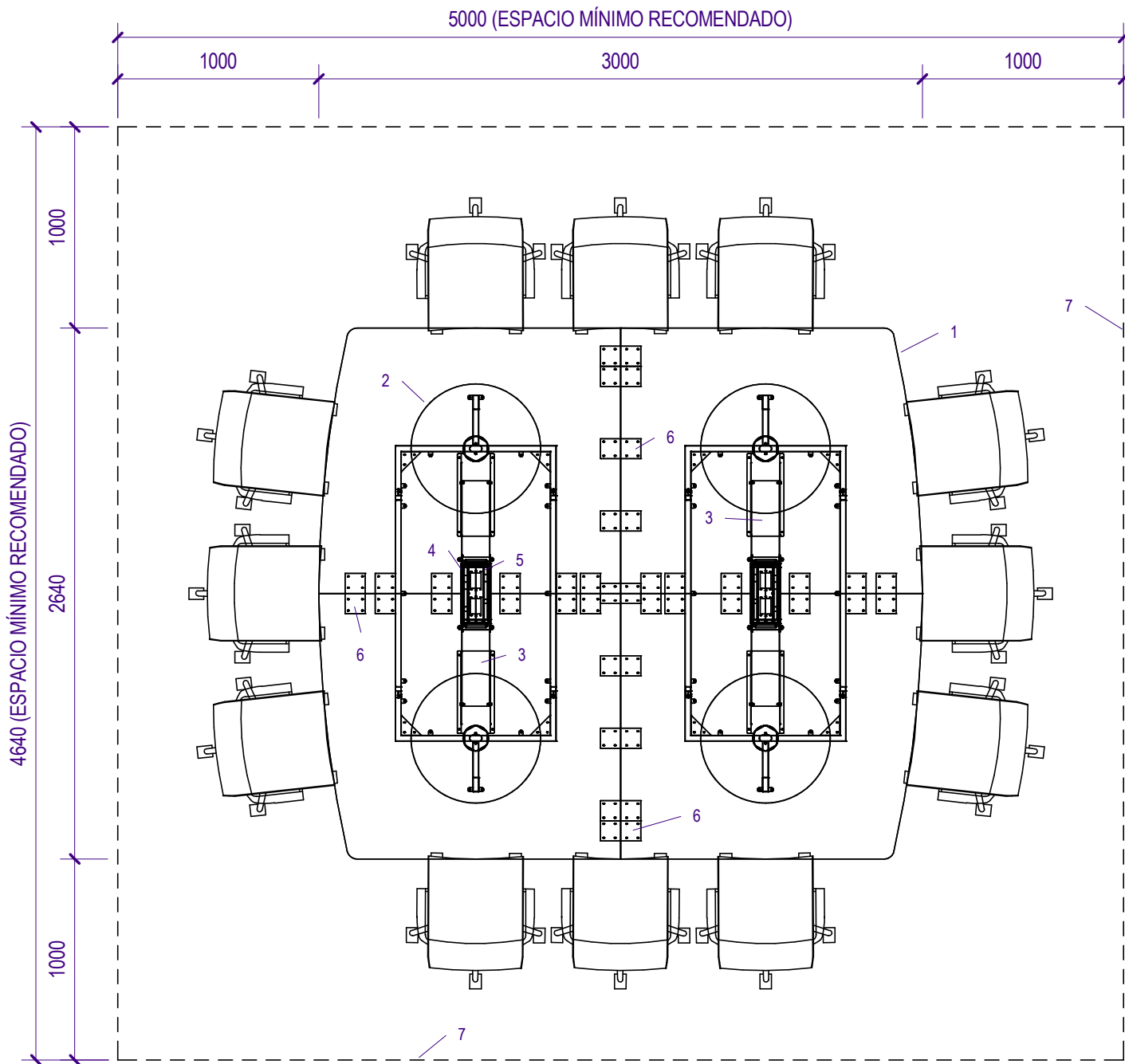
PLANTA TRANSPARENTE (ESCALA 1:30)
