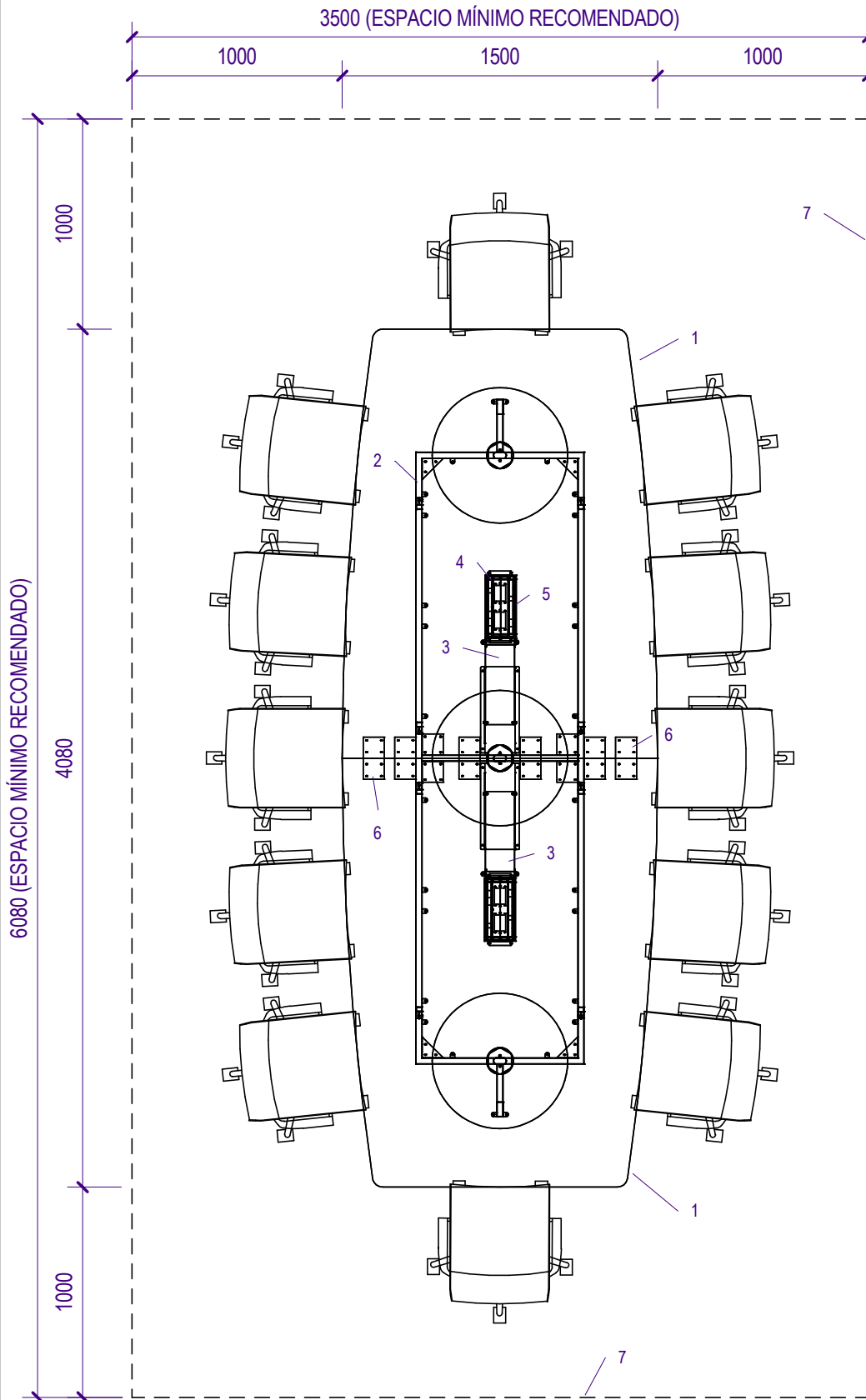
PLANTA TRANSPARENTE (ESCALA 1:30)
