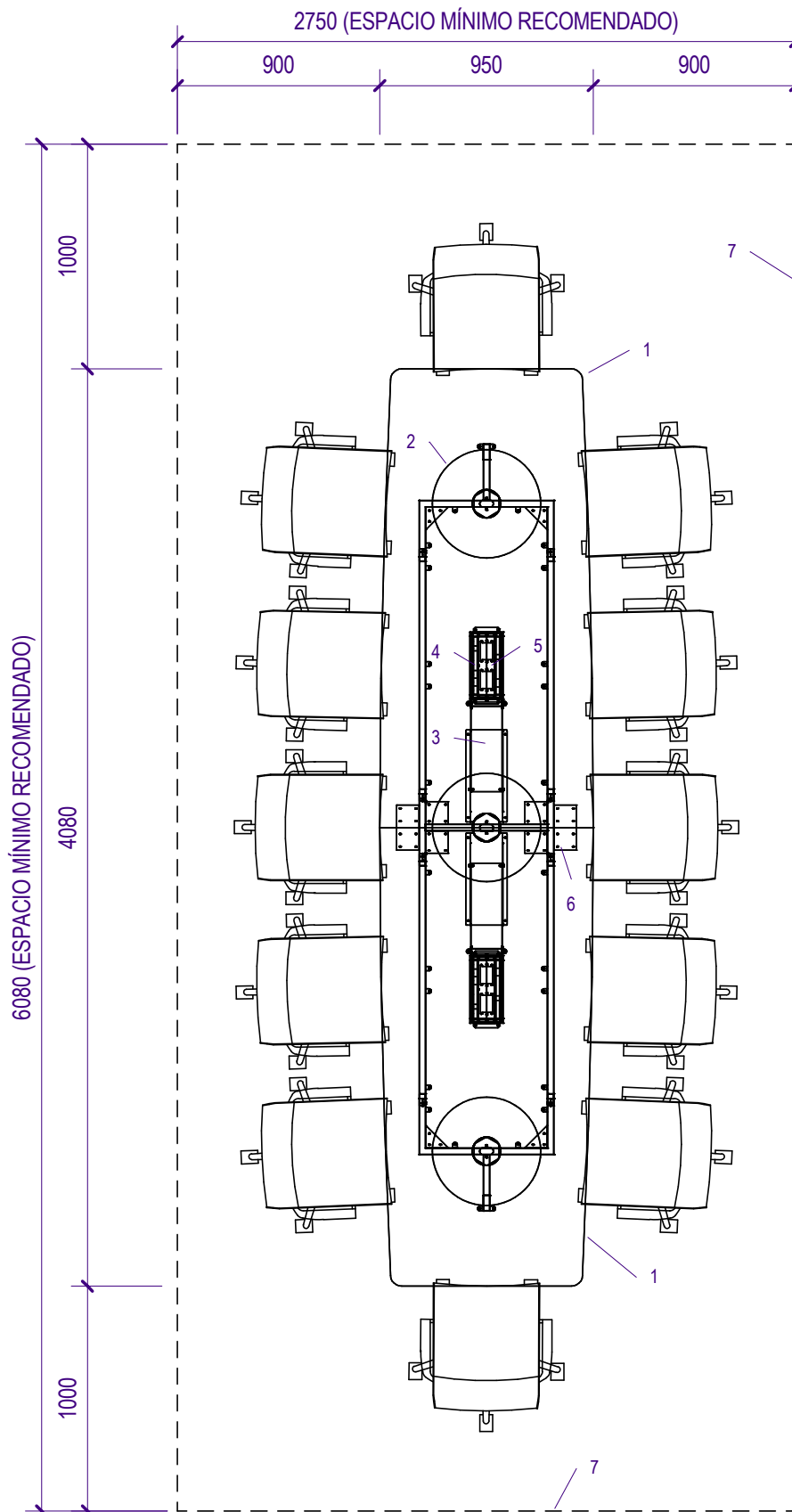
PLANTA TRANSPARENTE (ESCALA 1:30)
