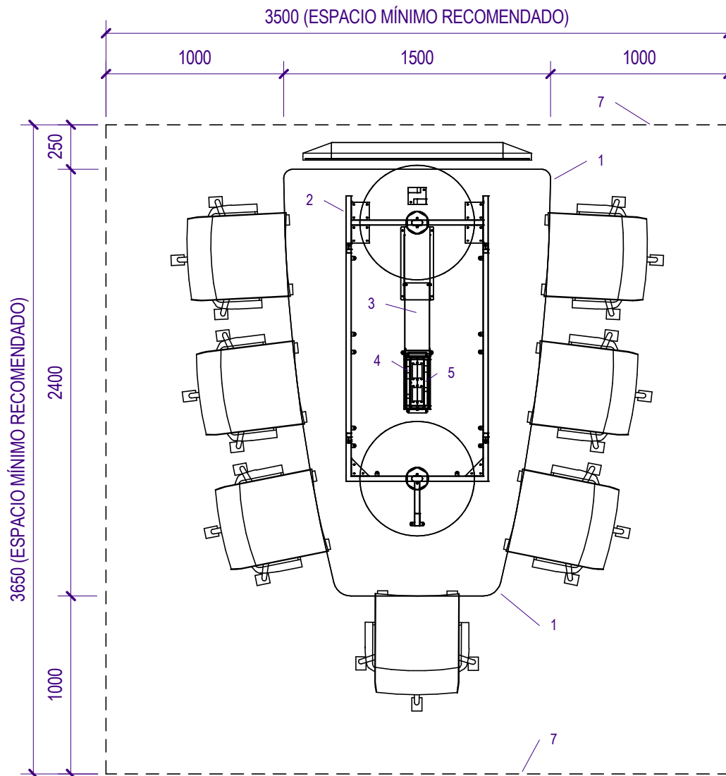
PLANTA TRANSPARENTE (ESCALA 1:30)
