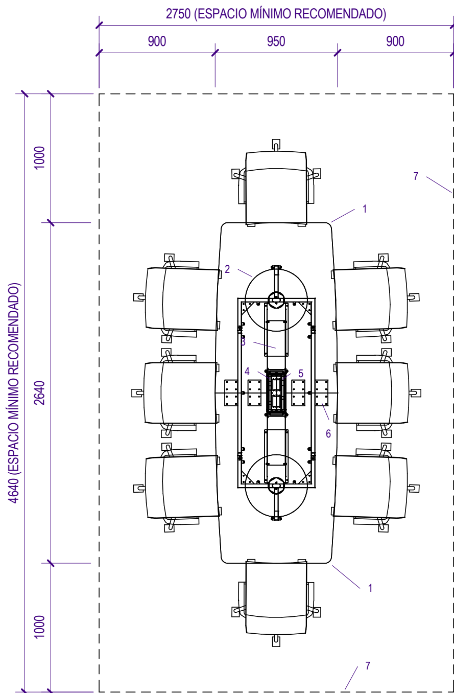
PLANTA TRANSPARENTE (ESCALA 1:30)
