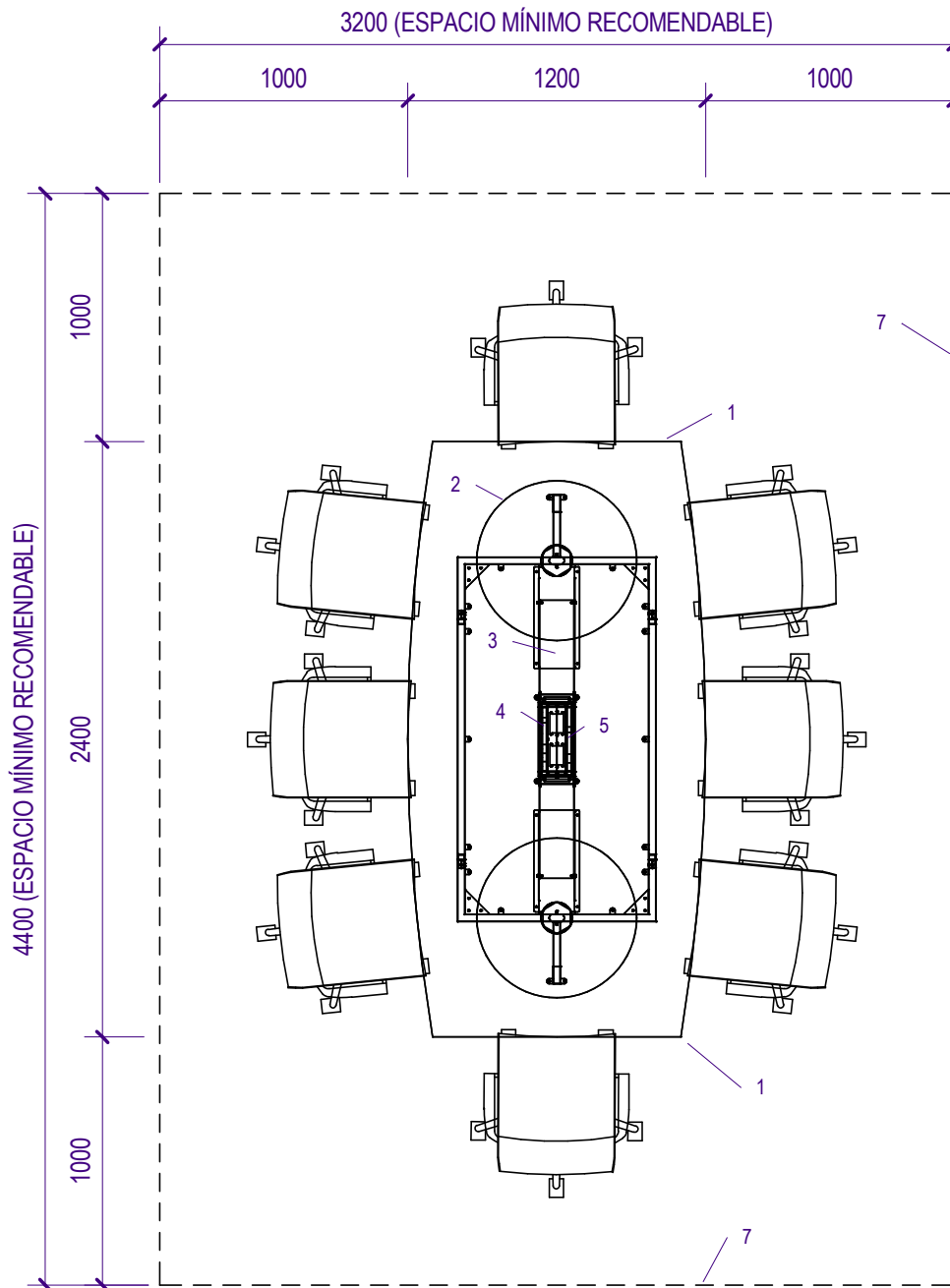
PLANTA TRANSPARENTE (ESCALA 1:30)
