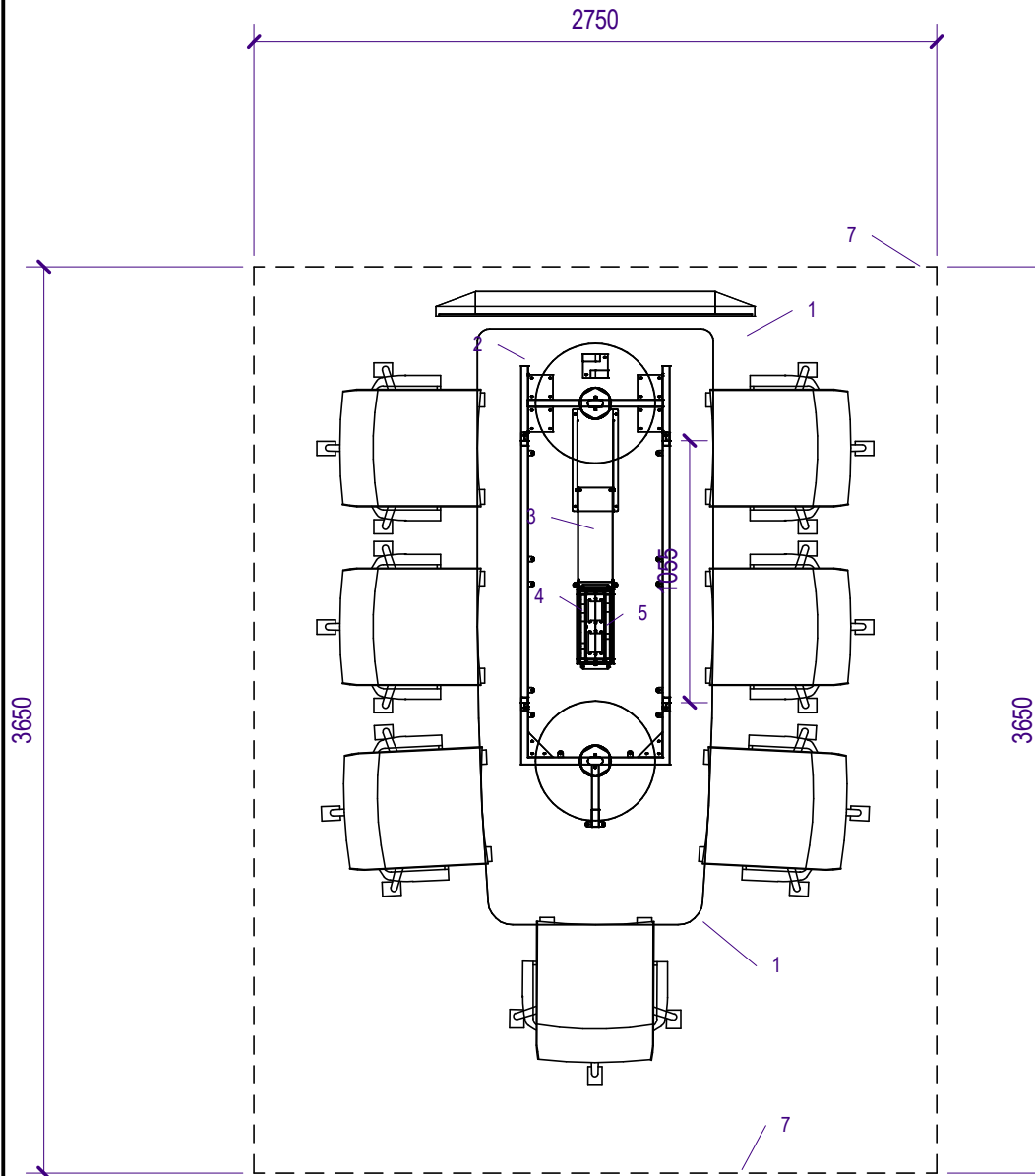
PLANTA TRANSPARENTE (ESCALA 1:30)
