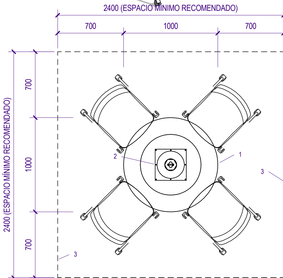
PLANTA TRANSPARENTE (ESCALA 1:25)
