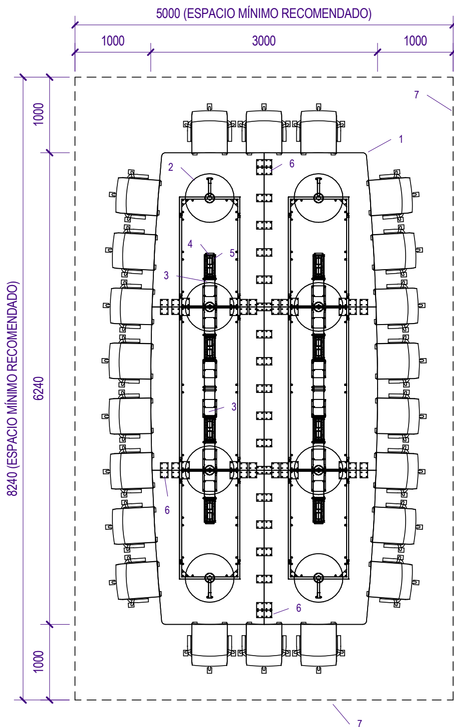
PLANTA TRANSPARENTE (ESCALA 1:50)
