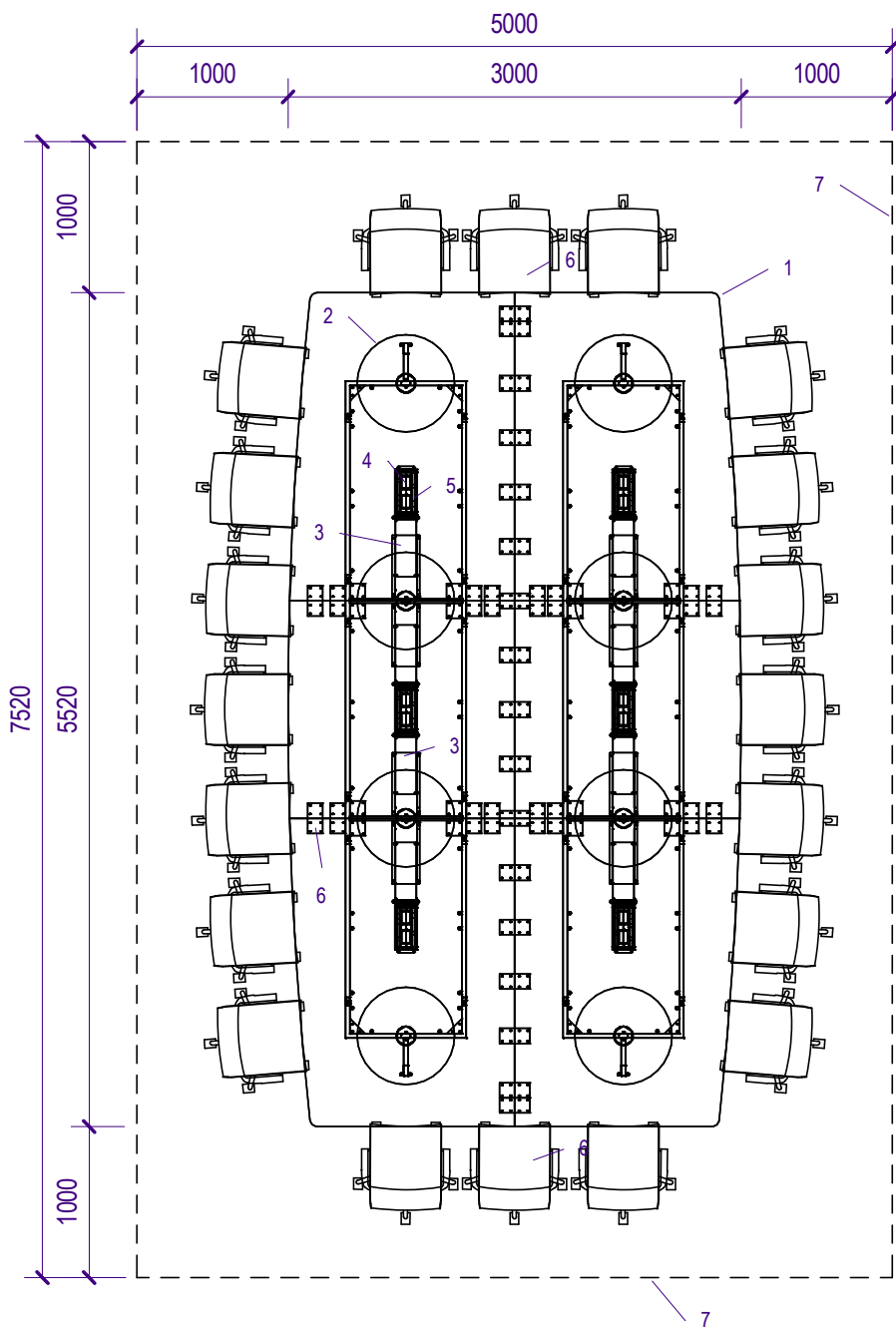
PLANTA TRANSPARENTE (ESCALA 1:50)
