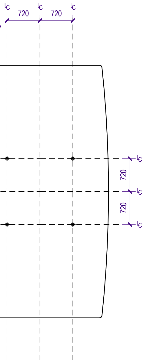
PLANTA DE CENTROS PARA ACOMETIDA DE CABLES
